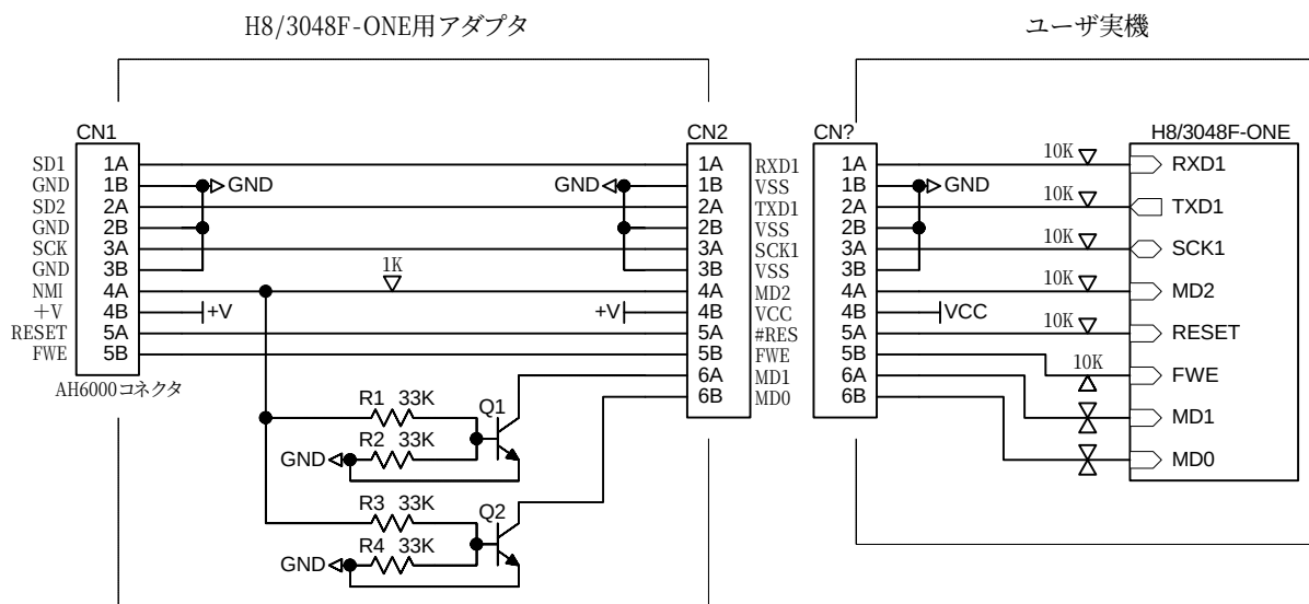
図2 E10Tコネクタとの互換性が無くてもよい場合
