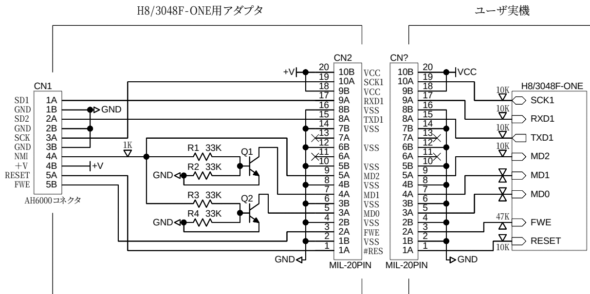
図1 E10Tのコネクタに合わせて製作する場合
