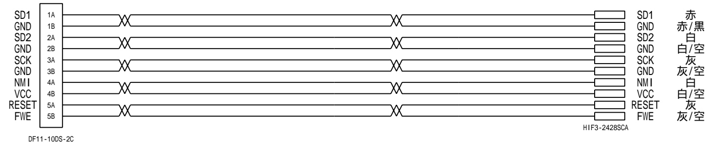
ケーブル結線図
