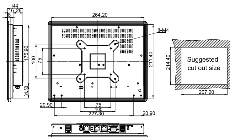
PPC-F10B-BT Dimensions (Unit: mm)
