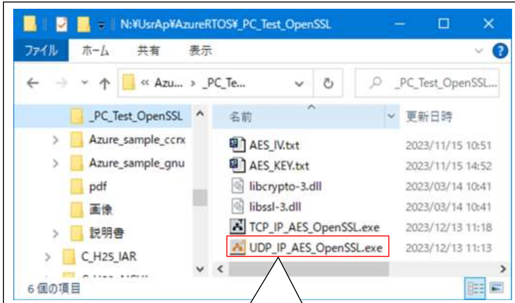
「UDP_IP_AES_OpenSSL.exe」を起動
