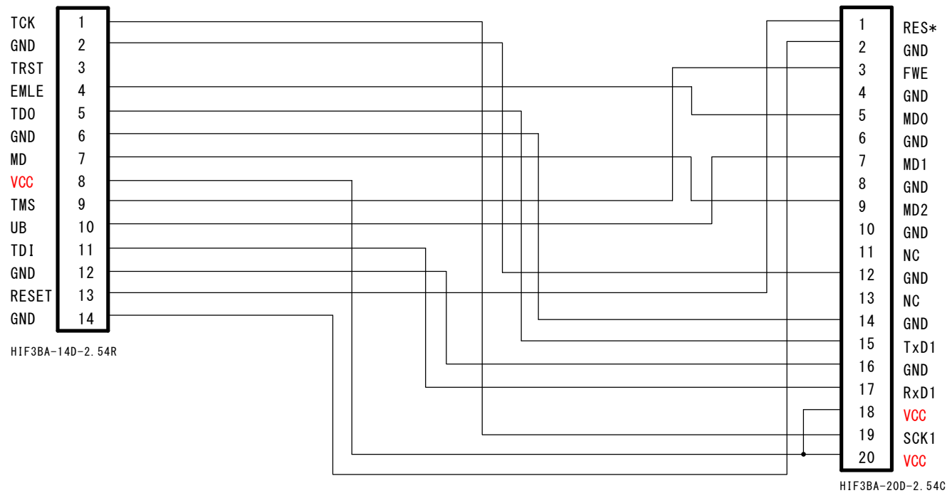
ケーブル結線図
